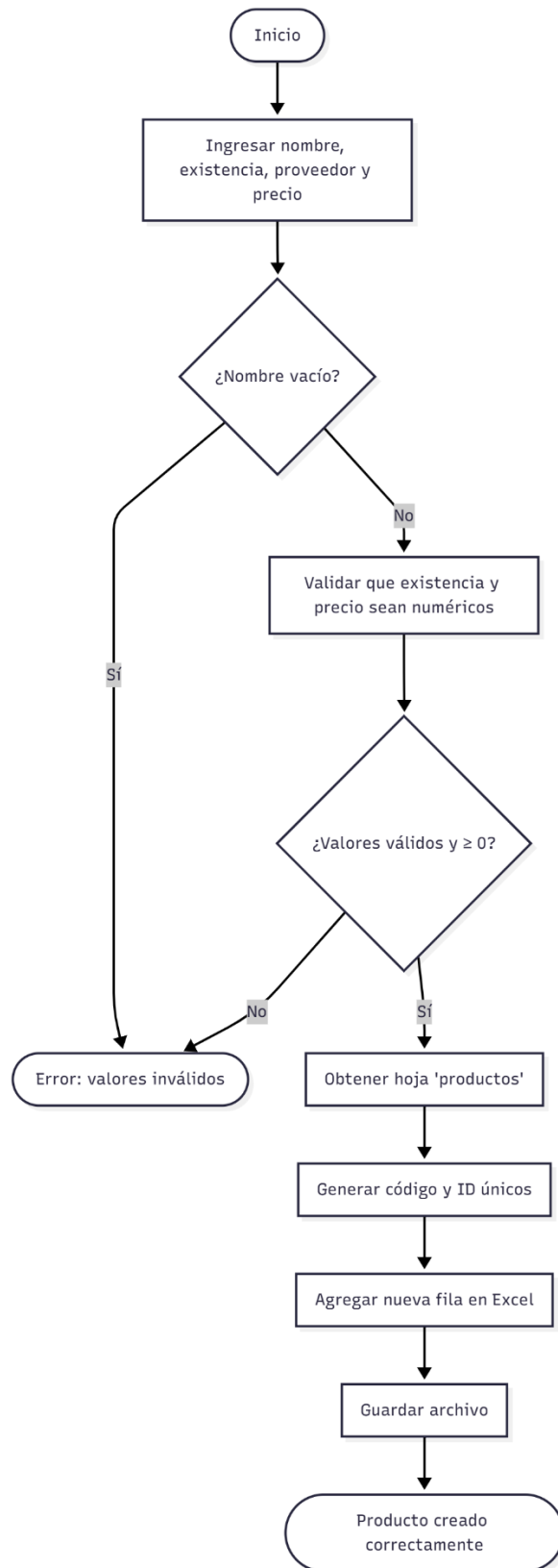
Diagrama de flujo “Crear Producto”
