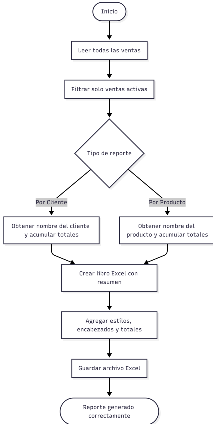
Diagrama de flujo “Generar Reporte por Cliente / Producto”
